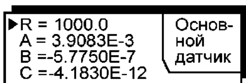
Рисунок 18 — Параметры ТСП
