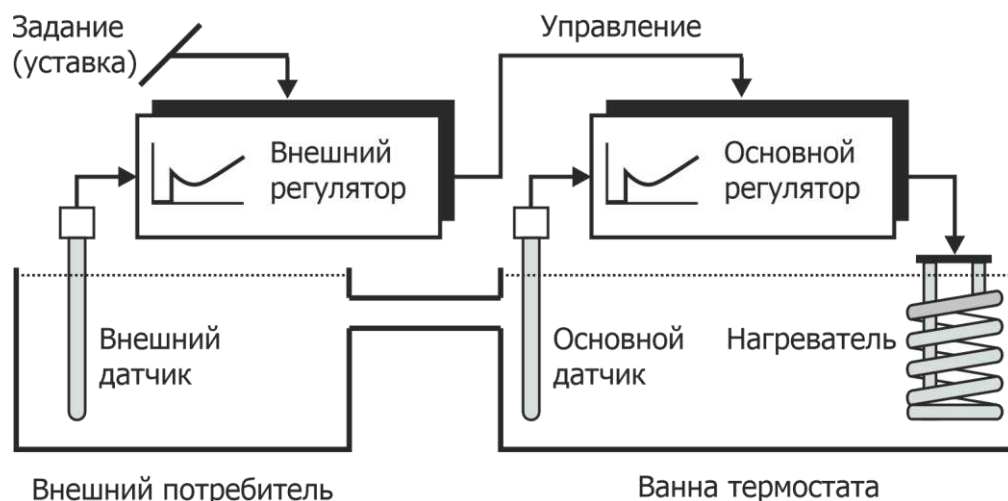
Рисунок 19 — Работа от внешнего датчика
