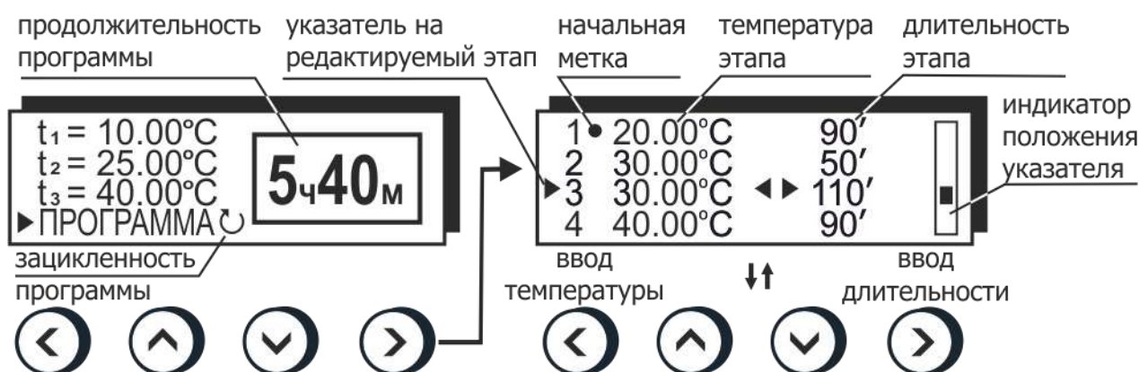
Рисунок 21 — Редактирование программы
